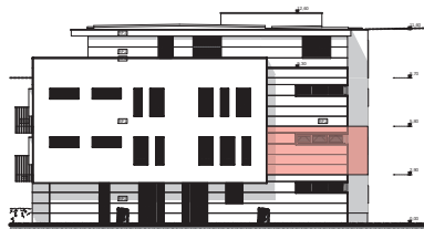
Façade Nord-Est
